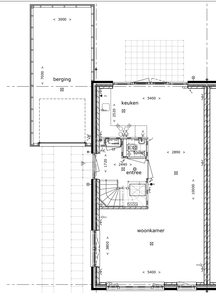
plattegrond begane grond optie vergrote berging
