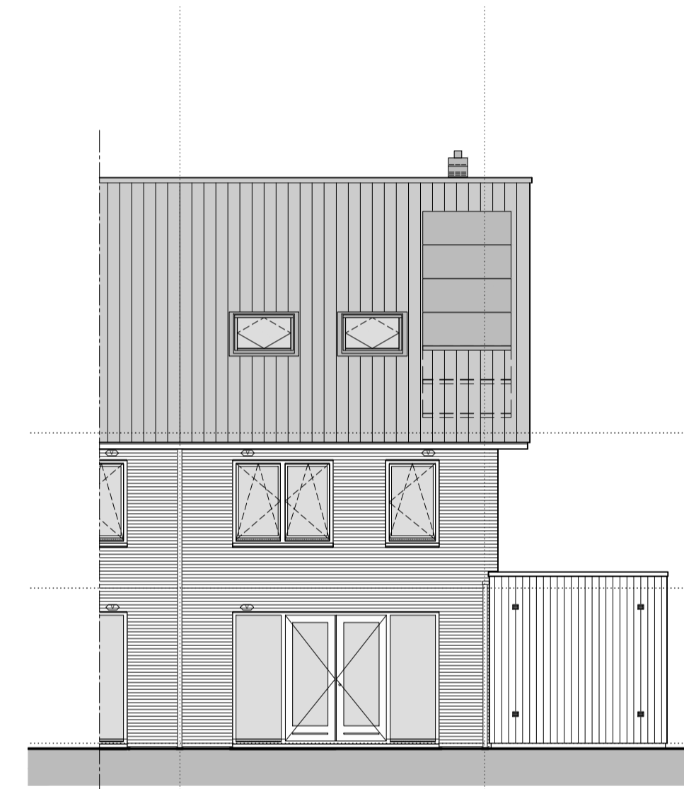
gevelaanzicht achtergevel optie dakvensters
