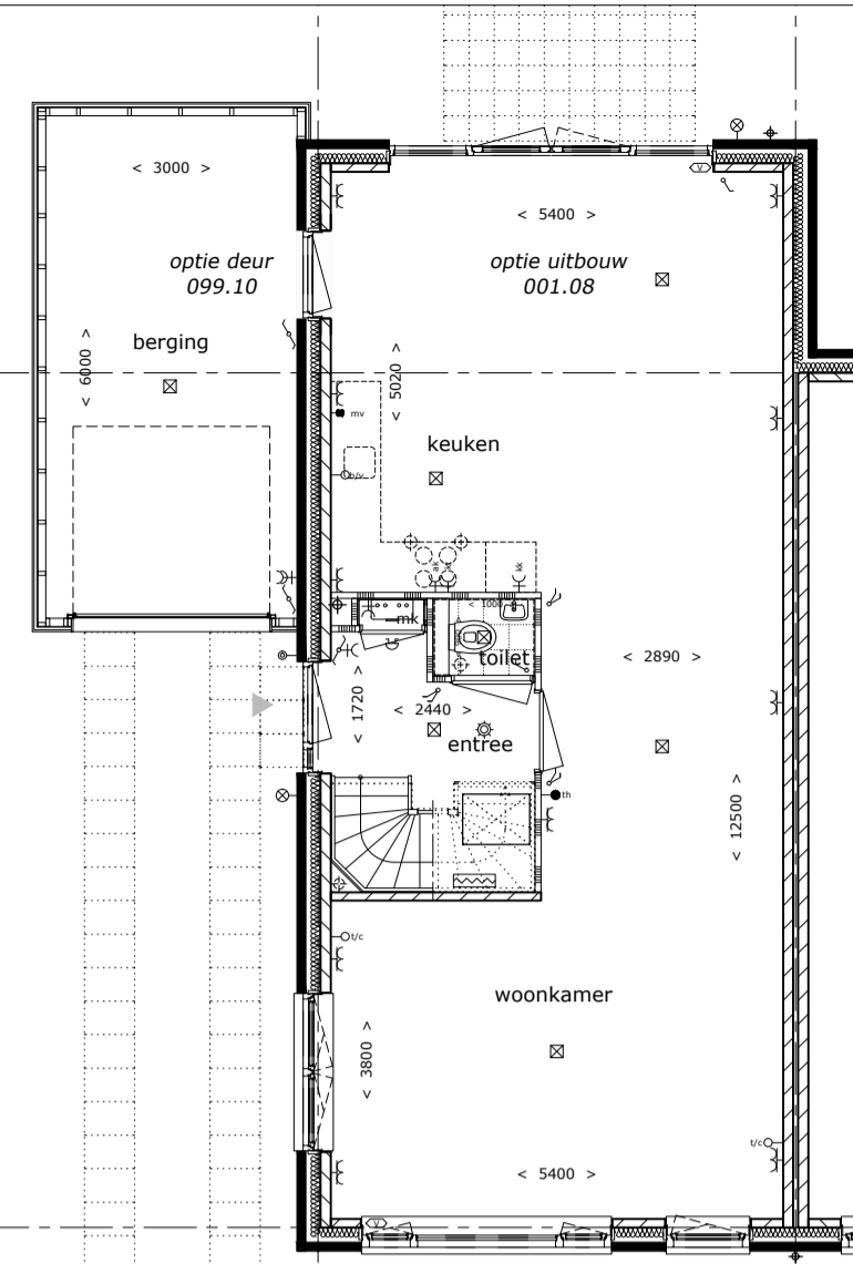
plattegrond begane grond optie uitbouw achterzijde
