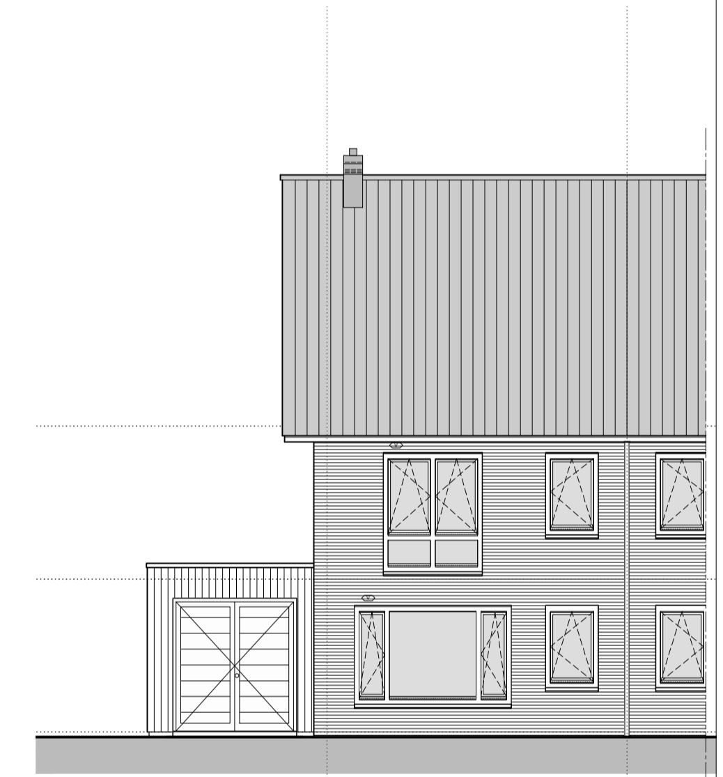
gevelaanzicht voorgevel optie dubbele deur berging
