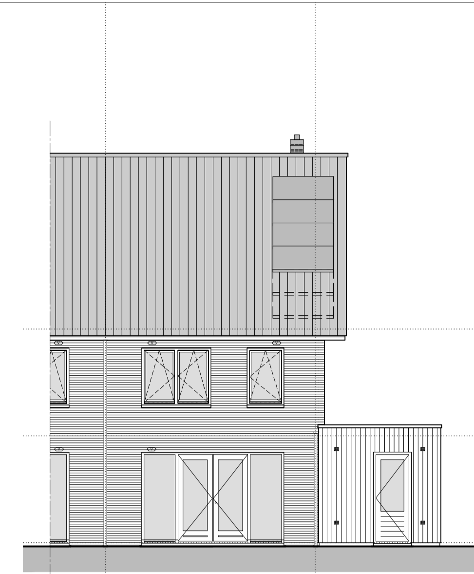
gevelaanzicht achtergevel optie deurkozijn berging
