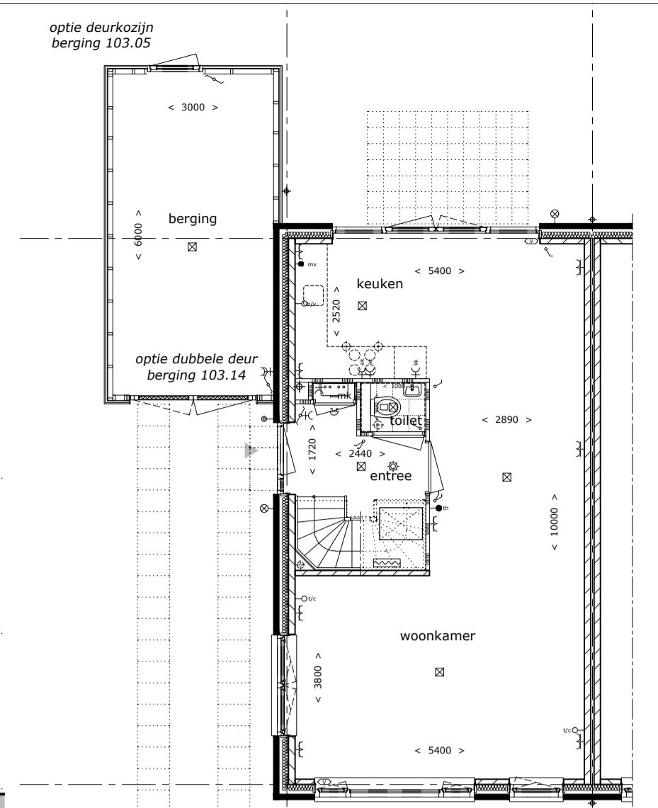
plattegrond begane grond optie kozijnen voor- en achterzijde
