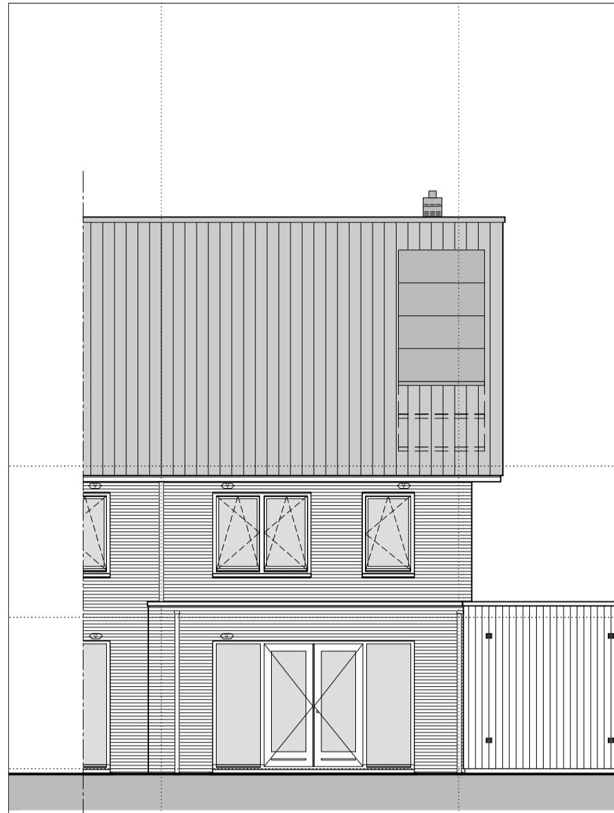
gevelaanzicht achtergevel optie uitbouw begane grond
