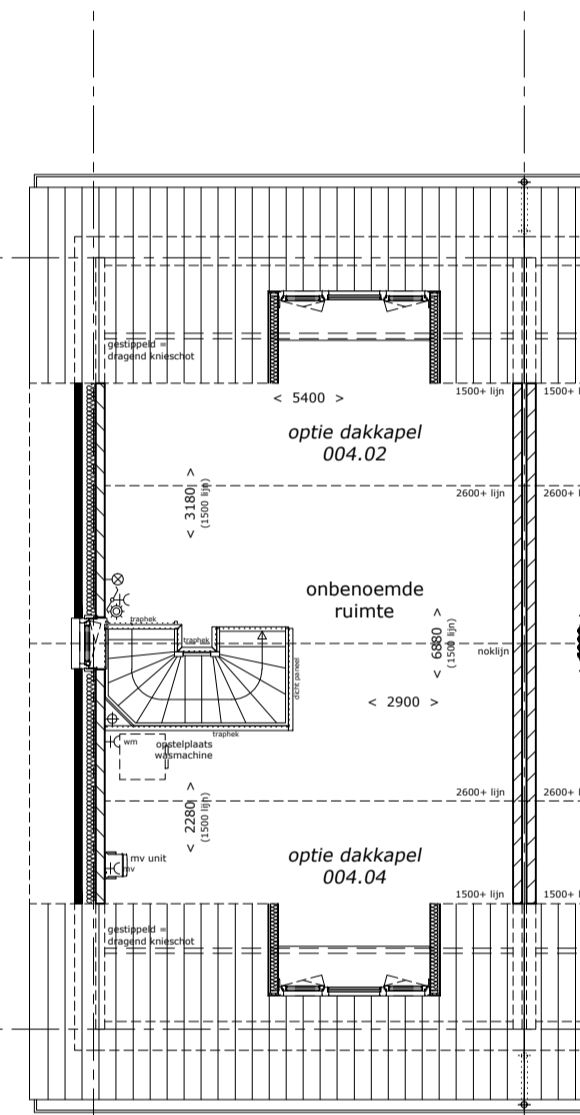
plattegrond 2e verdieping optie dakkapel voor- en/of achterzijde
