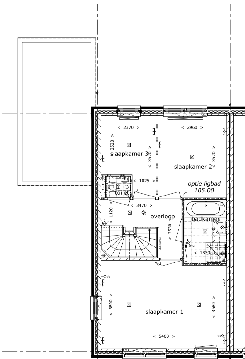
plattegrond 1e verdieping optie ligbad
