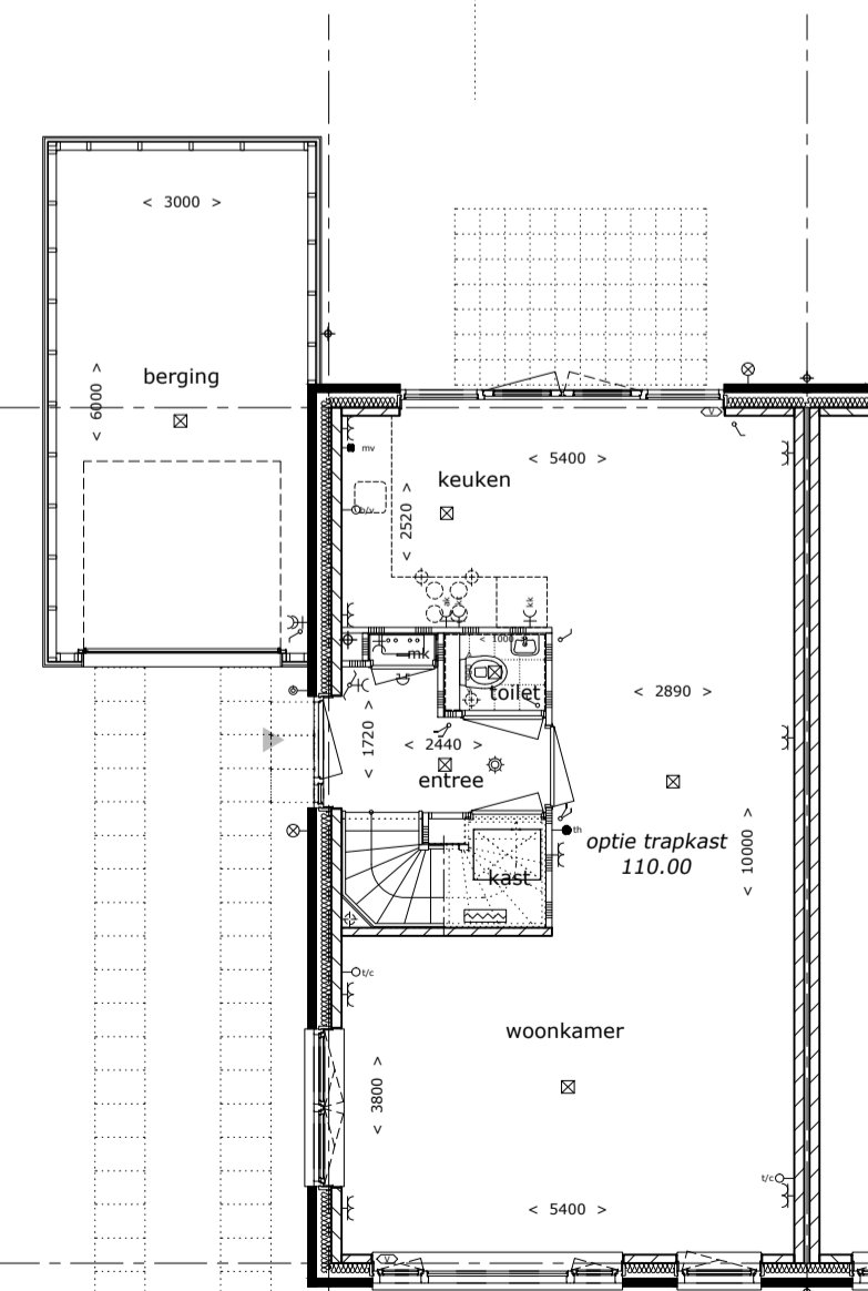
plattegrond begane grond optie trapkast
