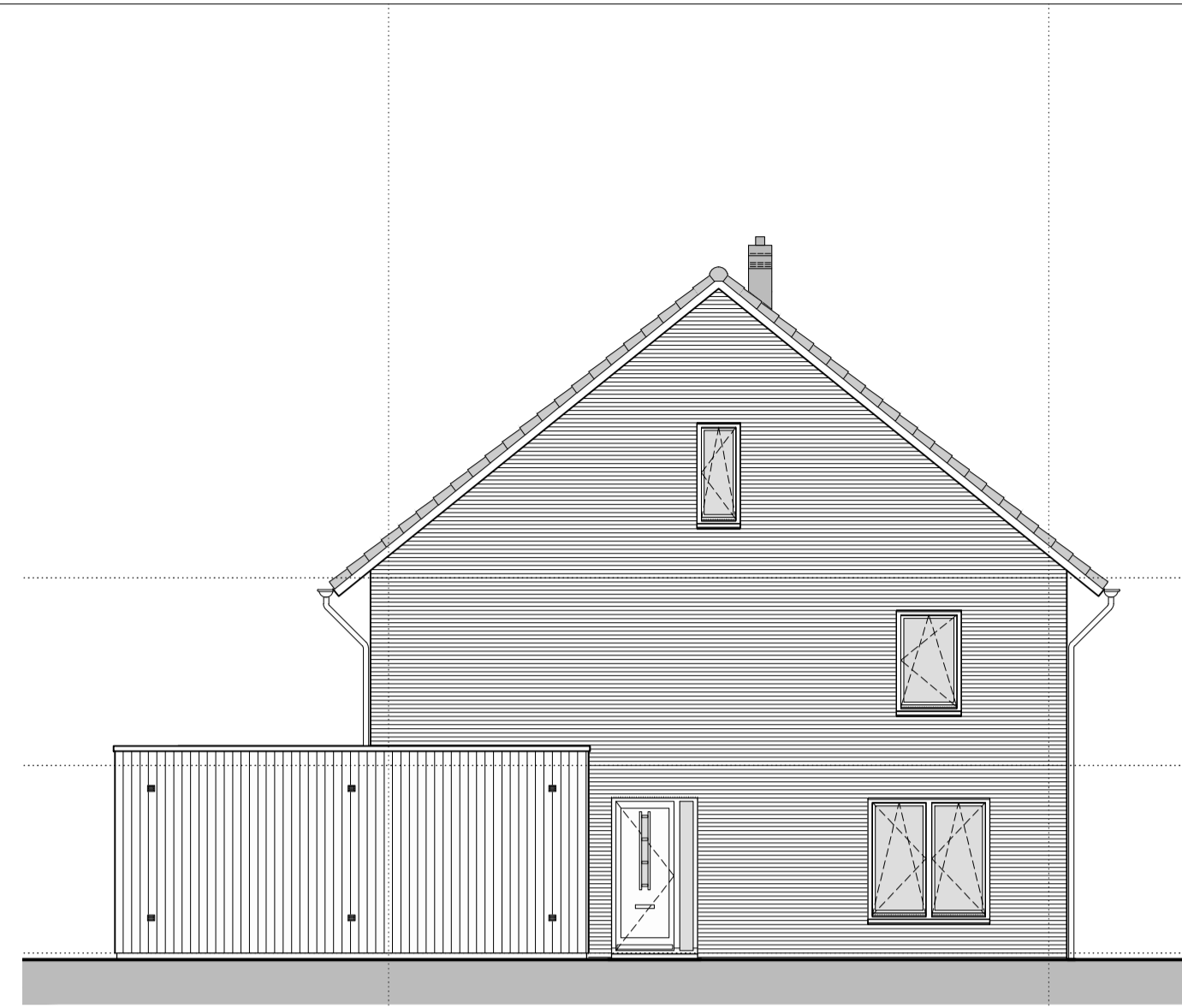
gevelaanzicht kopgevel vergrote berging
