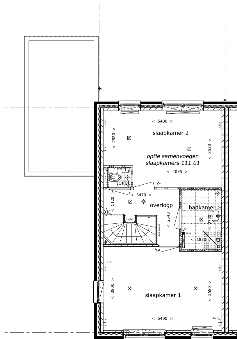
plattegrond 1e verdieping optie samenvoegen slaapkamers
