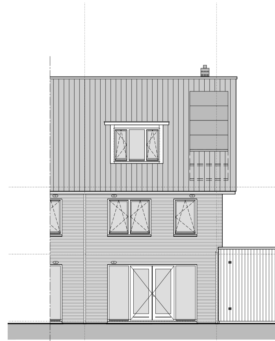
gevelaanzicht achtergevel optie dakkapel
