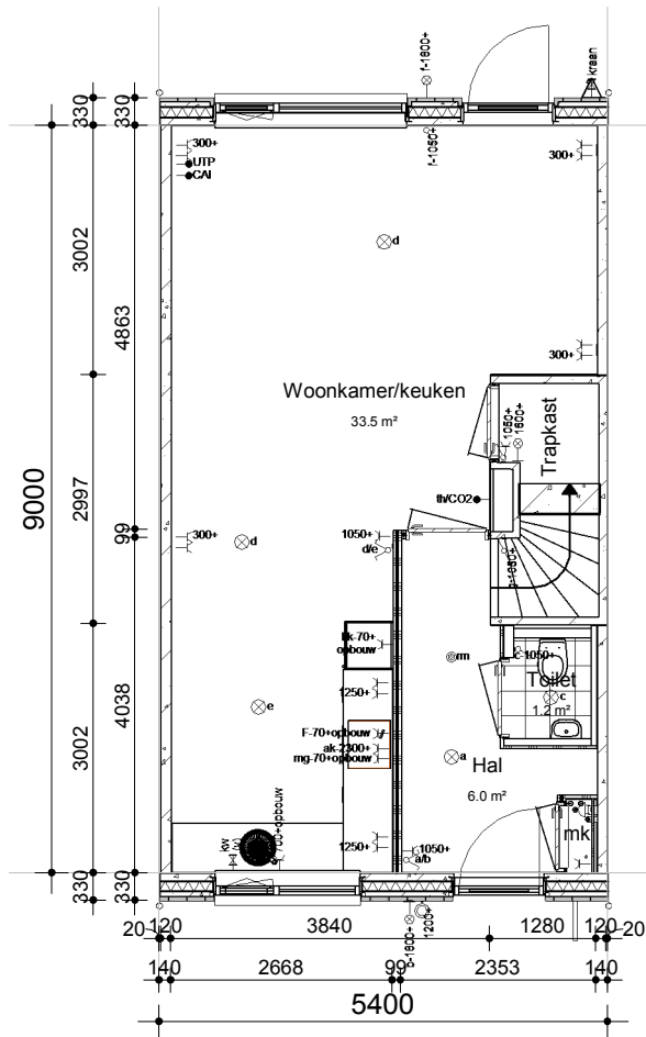
BEGANE GROND
