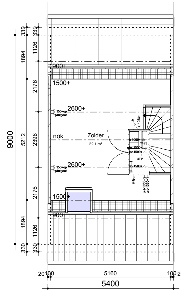
2de VERDIEPING
