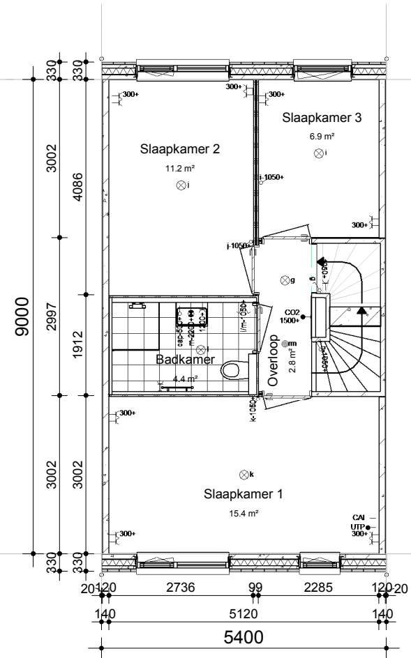
1e VERDIEPING
