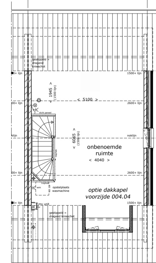
plattegrond 2e verdieping optie dakkapel voorzijde
