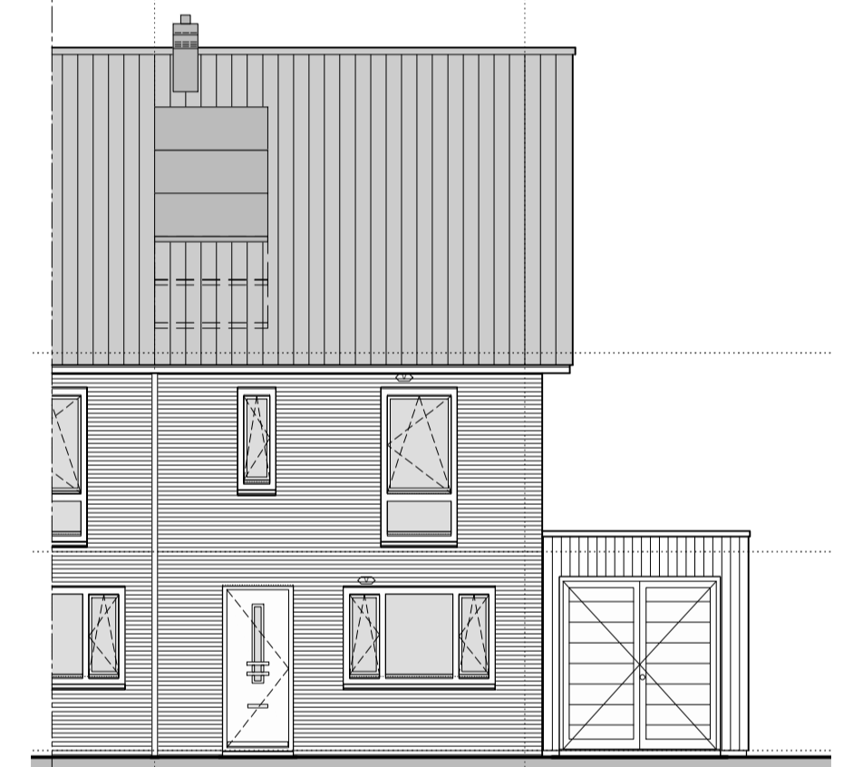
gevelaanzicht voorgevel optie dubbele deur berging
