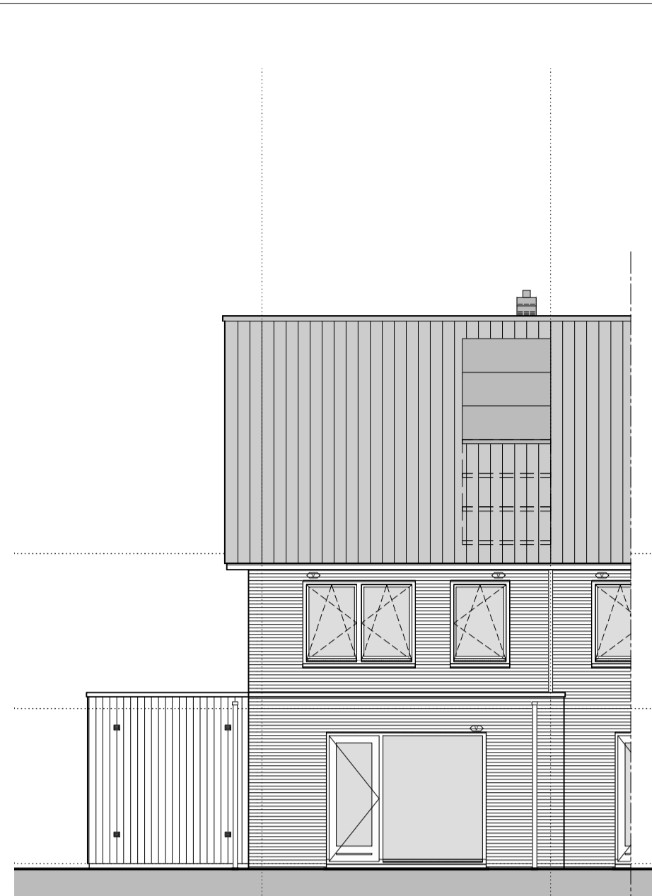
gevelaanzicht achtergevel optie uitbouw begane grond
