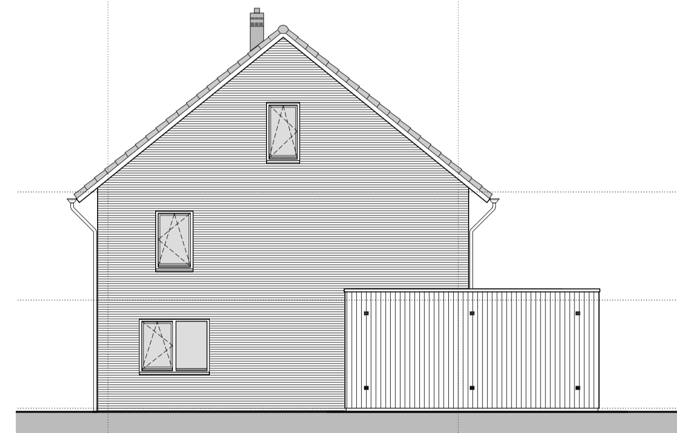
gevelaanzicht kopgevel vergrote berging
