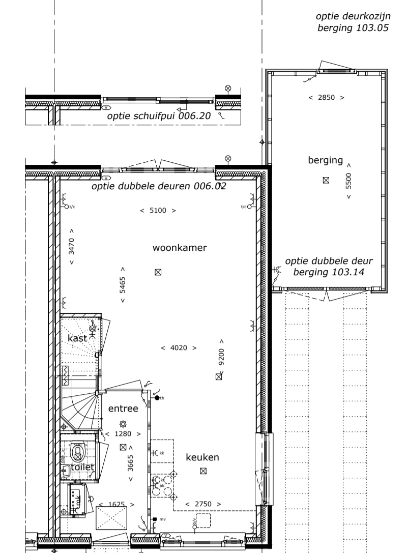
plattegrond begane grond optie kozijnen voor- en achterzijde
