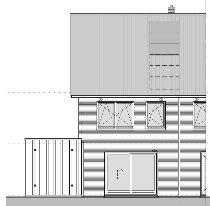
gevelaanzicht achtergevel optie schuifpui
