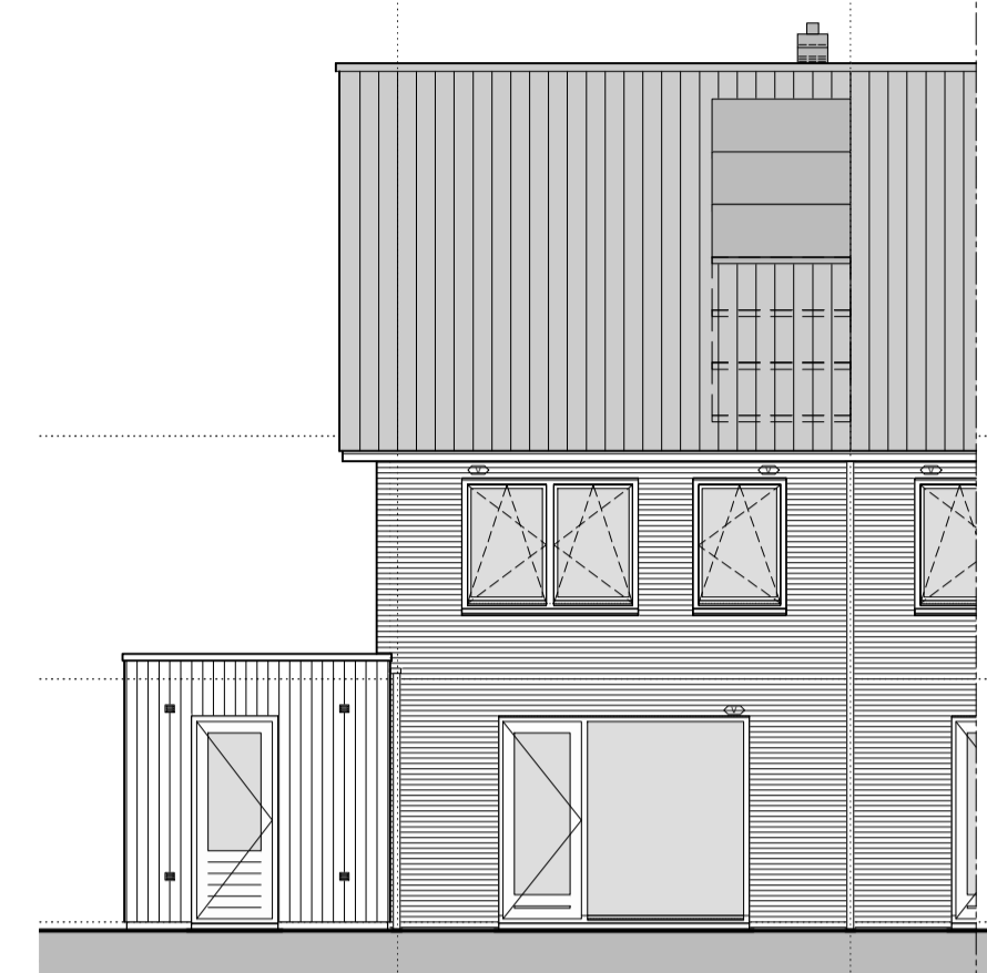
gevelaanzicht achtergevel optie deurkozijn berging
