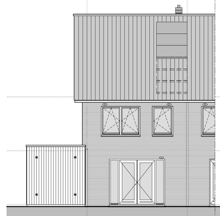
gevelaanzicht achtergevel optie dubbele deur
