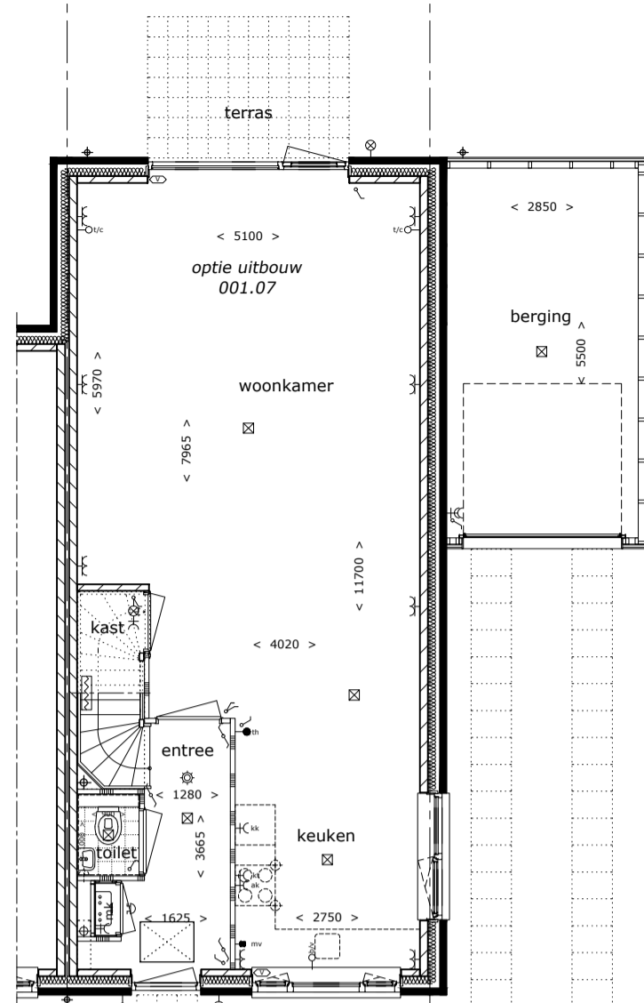
plattegrond begane grond optie uitbouw achterzijde
