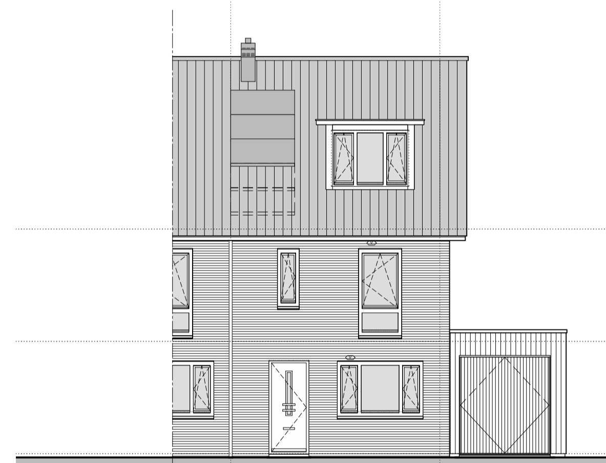
gevelaanzicht voorgevel optie dakkapel
