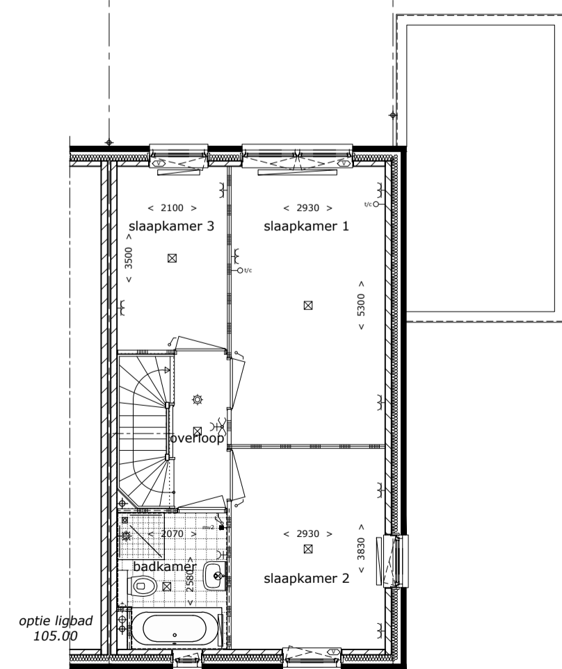
plattegrond 1e verdieping optie ligbad
