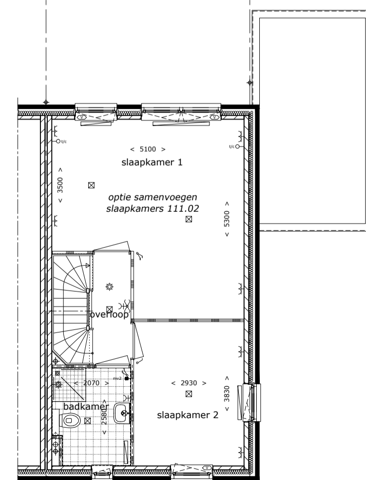
plattegrond 1e verdieping optie samenvoegen slaapkamers
