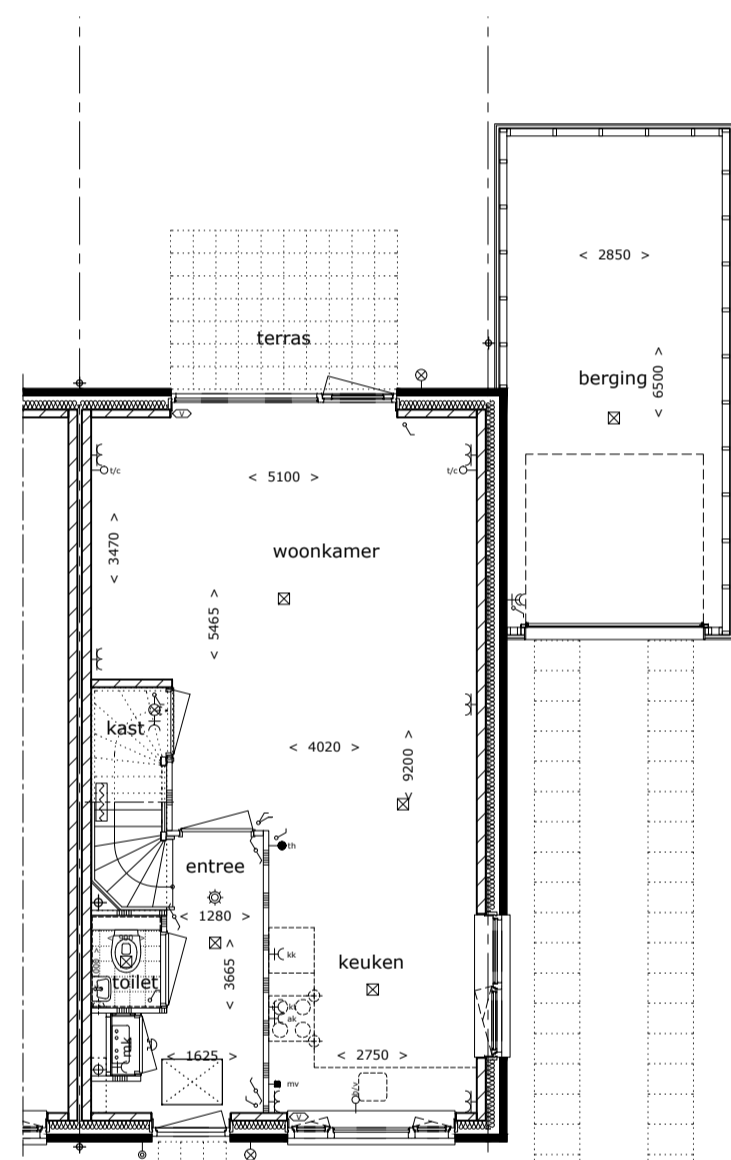
plattegrond begane grond optie vergrote berging
