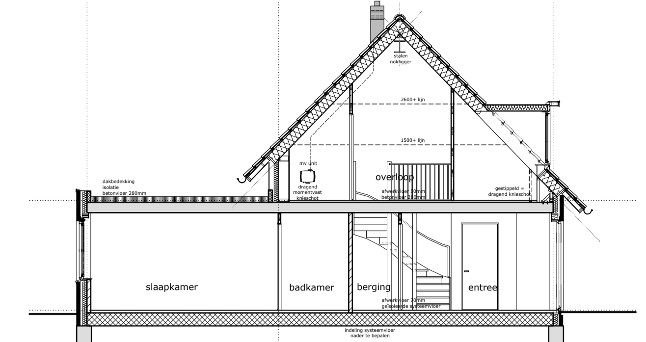
doorsnede
