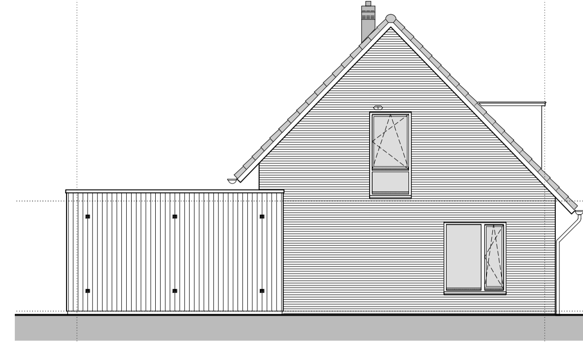
zijgevel
