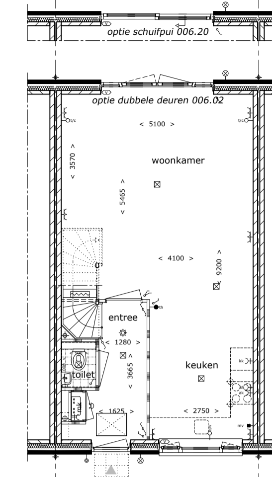
plattegrond begane grond optie kozijnen voor- en achterzijde
