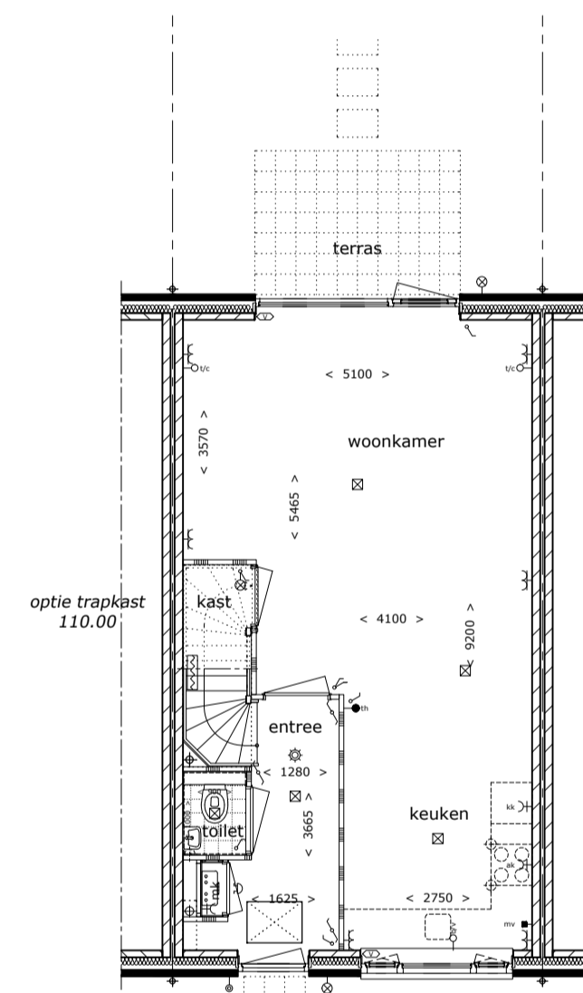
plattegrond begane grond optie trapkast
