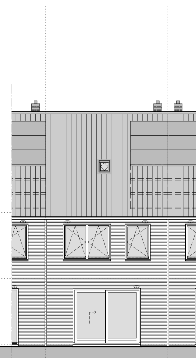
gevelaanzicht achtergevel optie schuifpui
