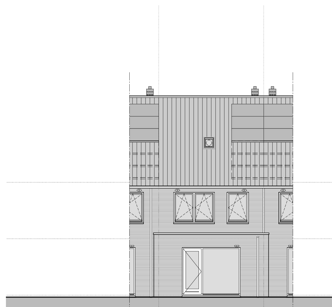
gevelaanzicht achtergevel optie uitbouw begane grond
