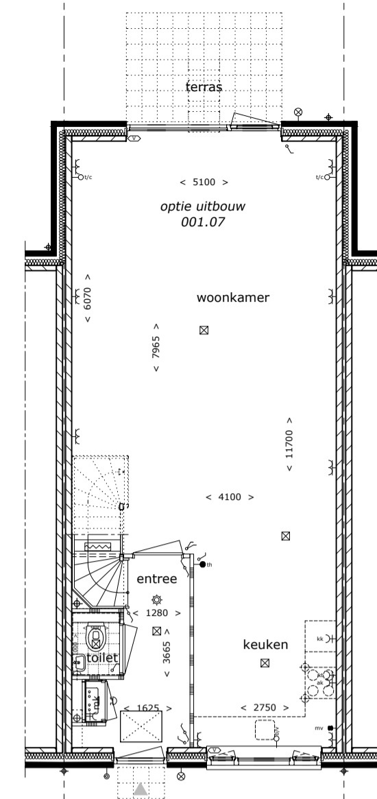
plattegrond begane grond optie uitbouw achterzijde
