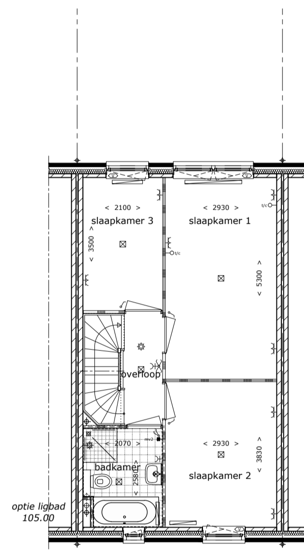
plattegrond 1e verdieping optie ligbad
