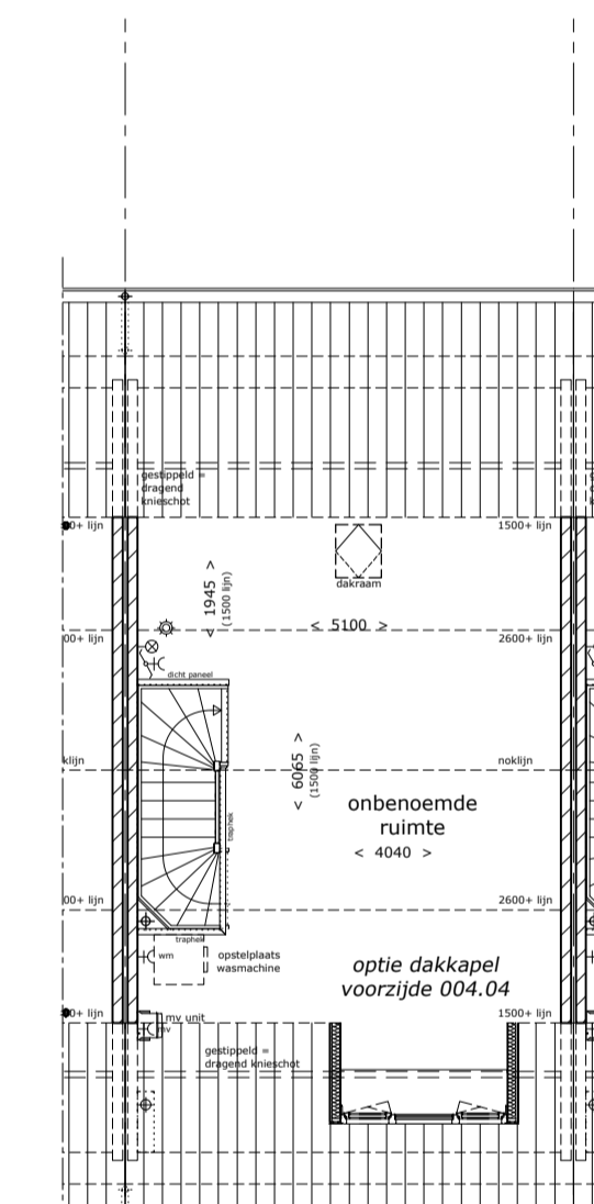
plattegrond 2e verdieping optie dakkapel voorzijde
