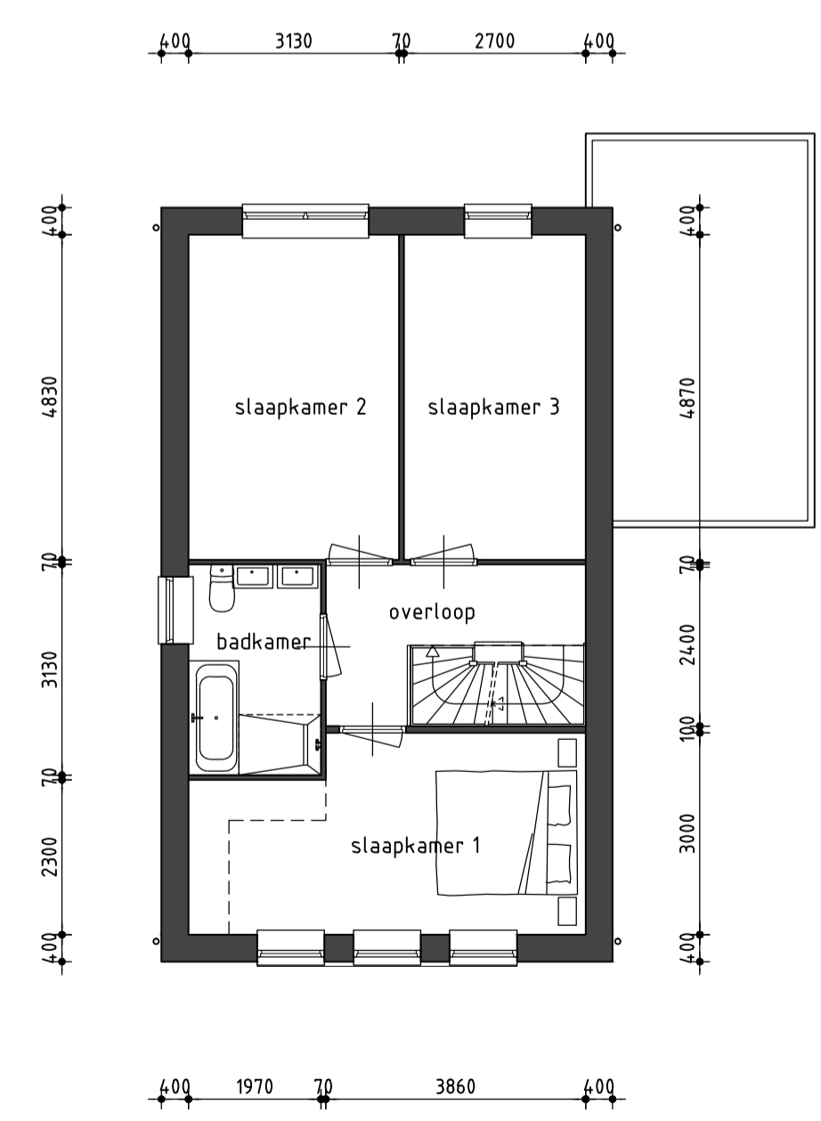
1e Verdieping
