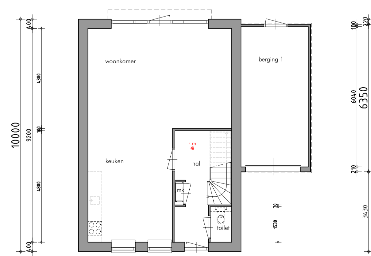
begane grond
