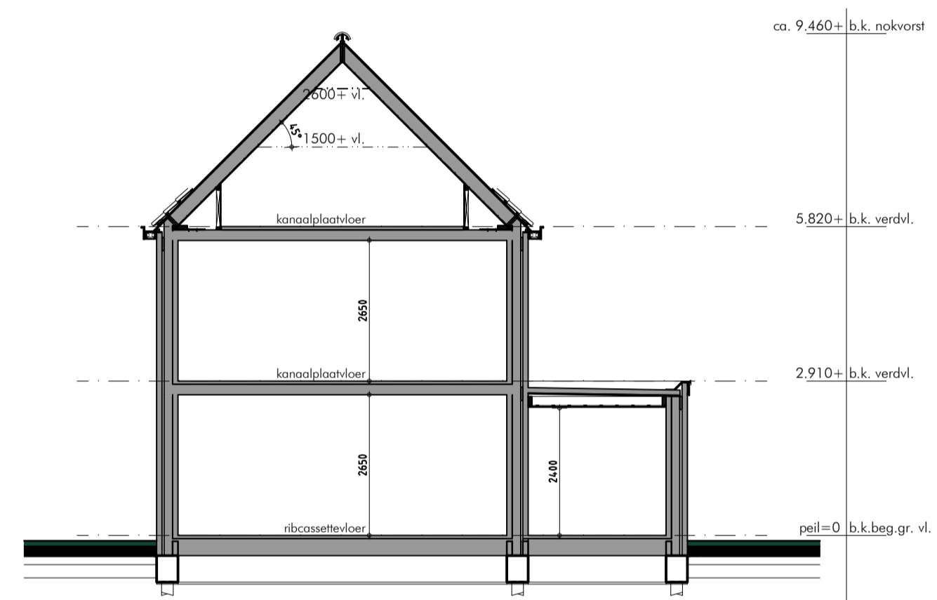
principe doorsnede
