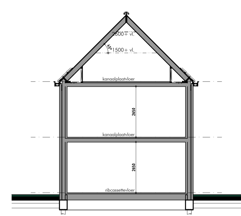
principe doorsnede
