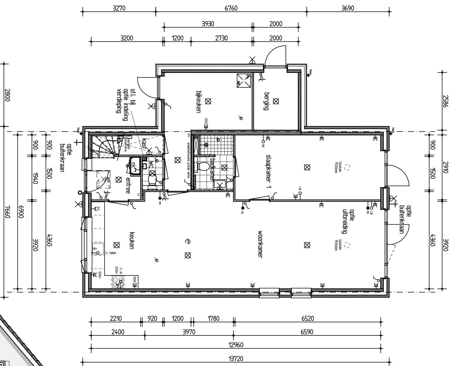
BEGANE GROND
