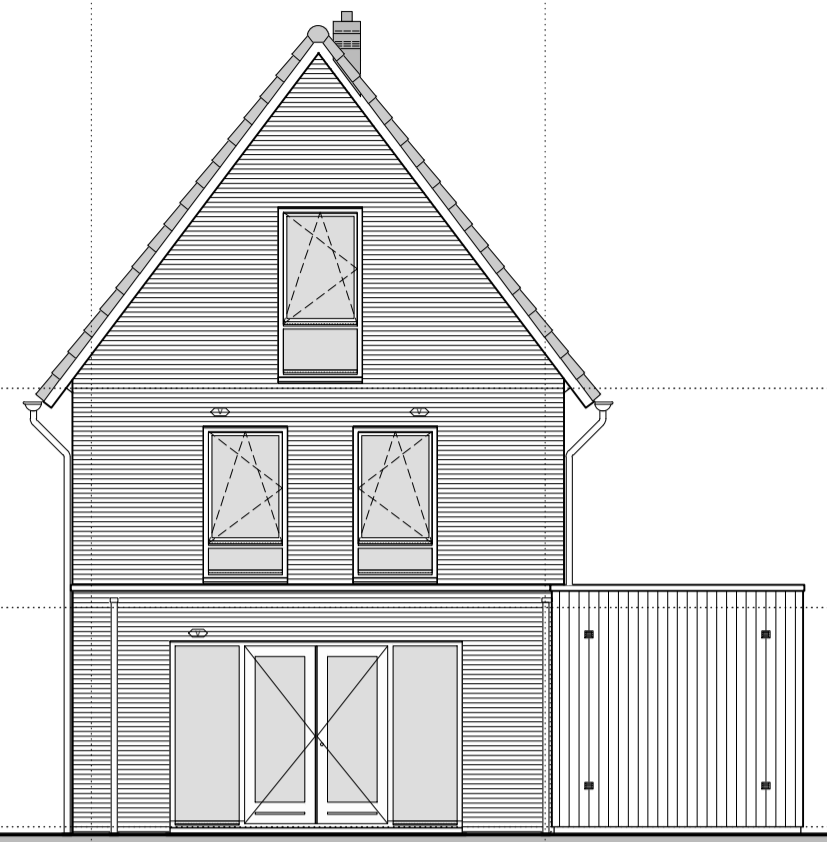
gevelaanzicht achtergevel optie uitbouw begane grond
