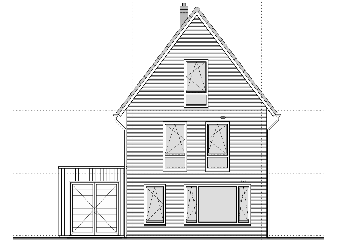
gevelaanzicht voorgevel optie dubbele deur berging
