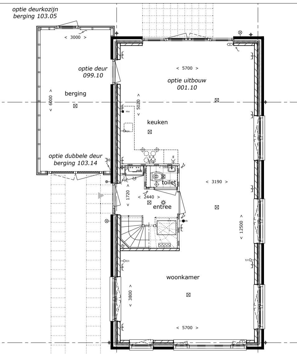
plattegrond begane grond optie uitbouw en optie gevelkozijnen
