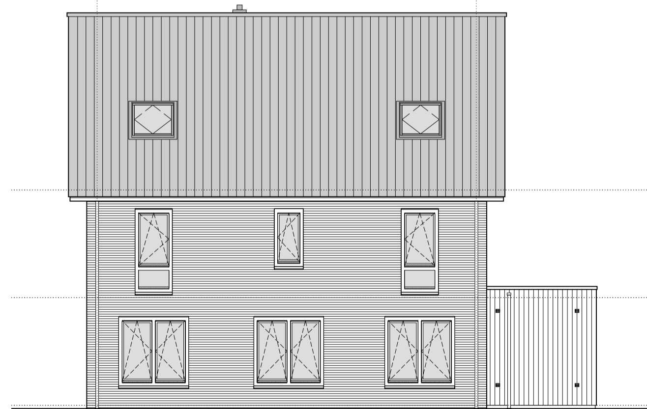
gevelaanzicht zijgevel straatzijde optie dakvensters
