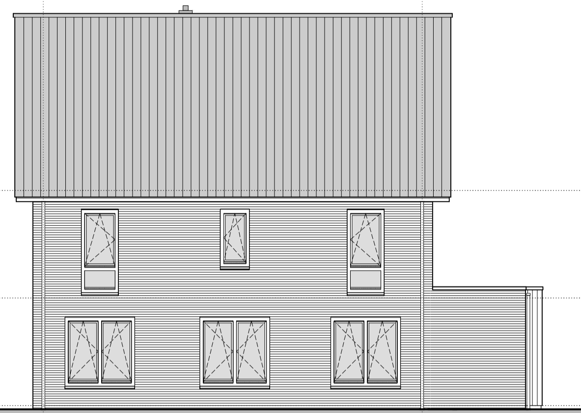
gevelaanzicht zijgevel tuinzijde optie uitbouw
