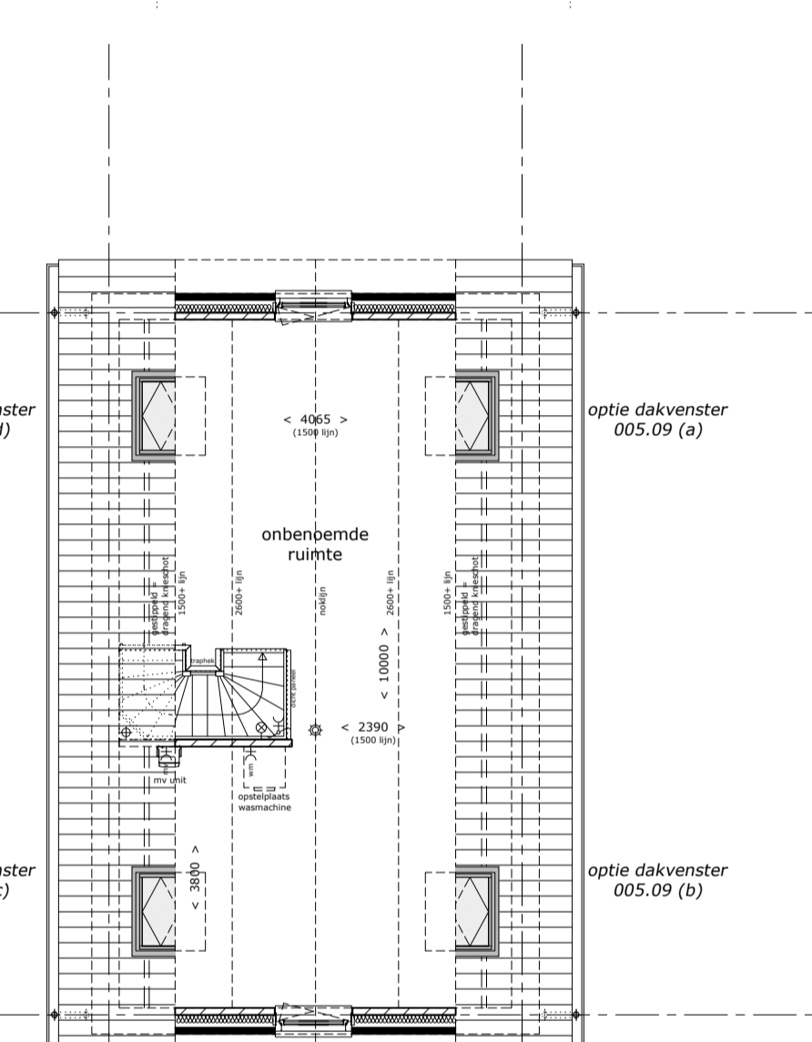
plattegrond 2e verdieping optie dakvensters
