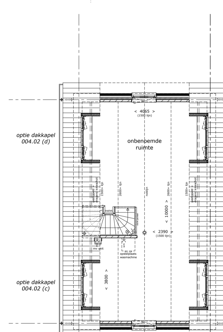
plattegrond 2e verdieping optie dakkapellen
