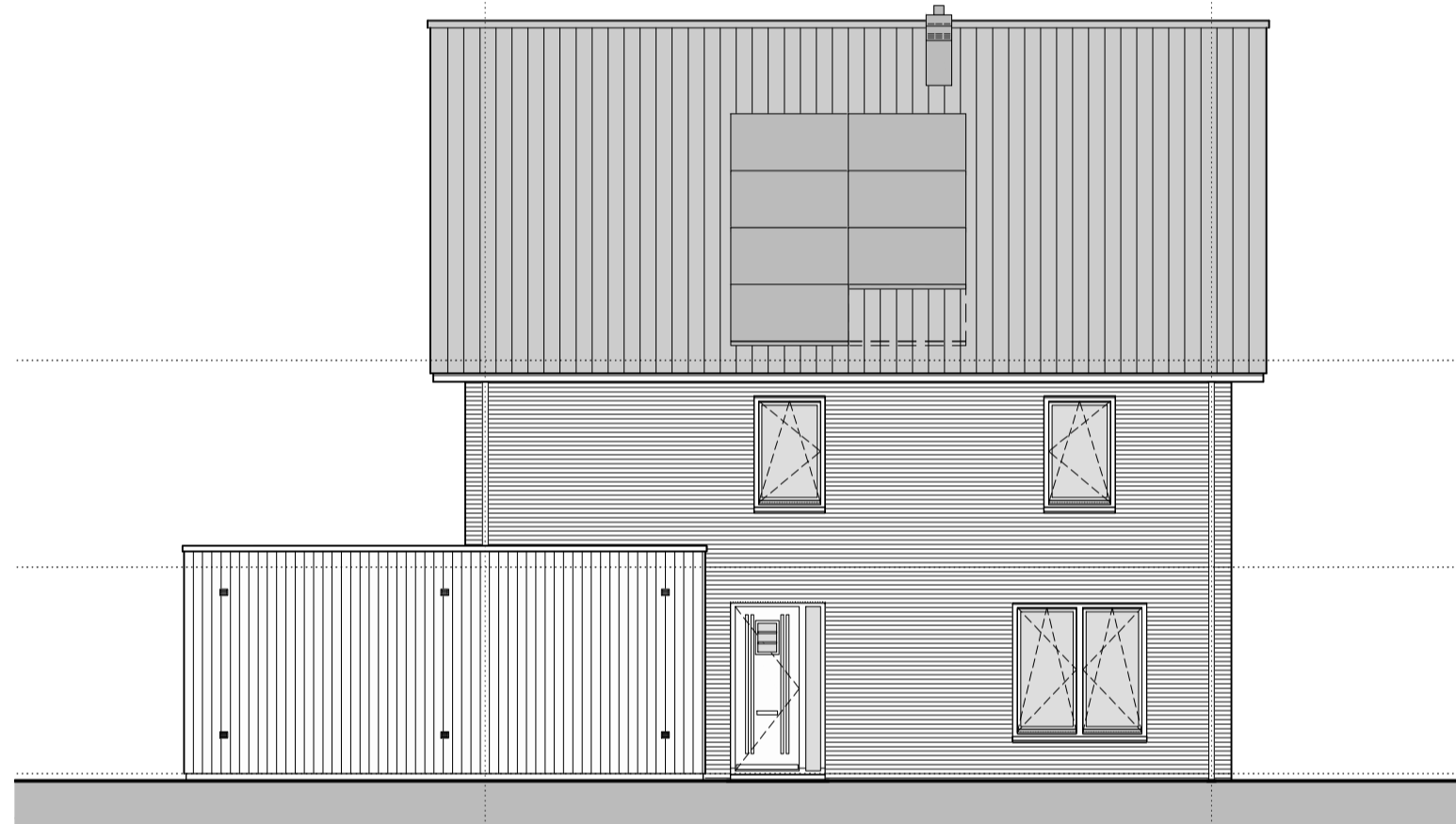
gevelaanzicht zijgevel entreezijde optie vergrote berging
